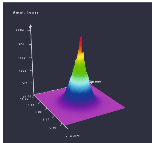
BM+ による出力密度分布の測定
