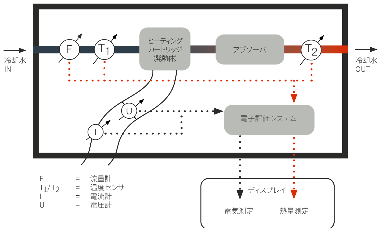
ECパワーモニタ 基準測定の原理
